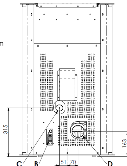
Dimensions du poêle à granulés AURORA
