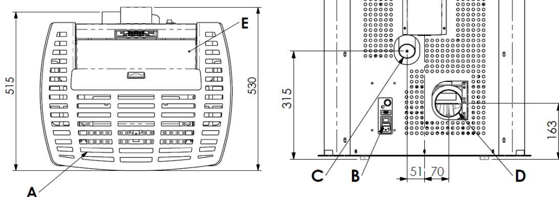
Ingombri stufa pellet AURORA
